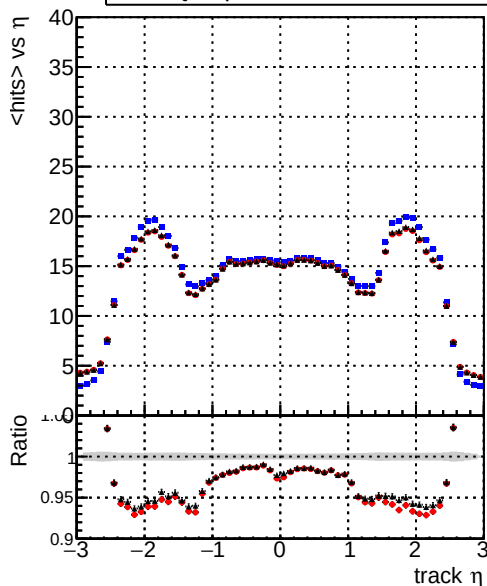
mean hits — DQMstep3_TT_CKF — DQMstep3_TT_default — DQMstep3_TT_ckfPixelLess
