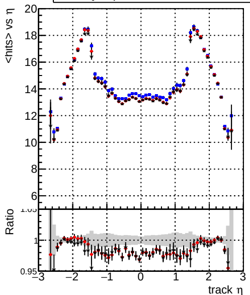
mean hits — DQMstep3 TT_CKF — DQMstep3 TT_CKF-t00 — DQMstep3 TT_CKF-t01
