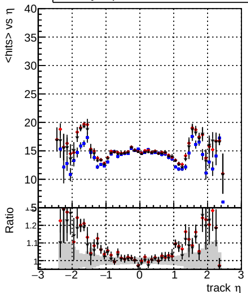
mean hits — DQMstep3_TT_CKF — DQMstep3_TT_CKF-t00 — DQMstep3_TT_CKF-t01
