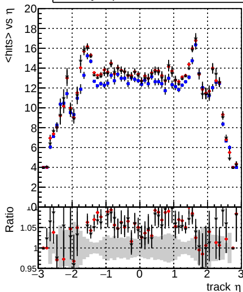
mean hit — DQMstep3_TT_CKF — DQMstep3_TT_CKF-t00 — DQMstep3_TT_CKF-t01
