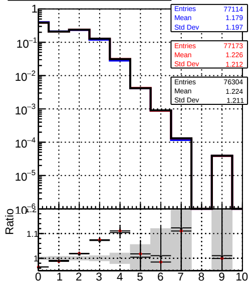
mean hits — DQMstep3_TT_CKF — DQMstep3_TT_CKF-t00 — DQMstep3_TT_CKF-t01
