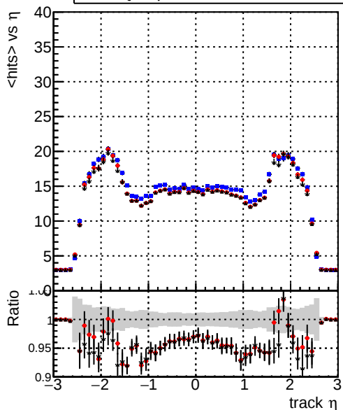
mean hits — DQMstep3_TT_CKF — DQMstep3_TT_CKF-t00 — DQMstep3_TT_CKF-t01
