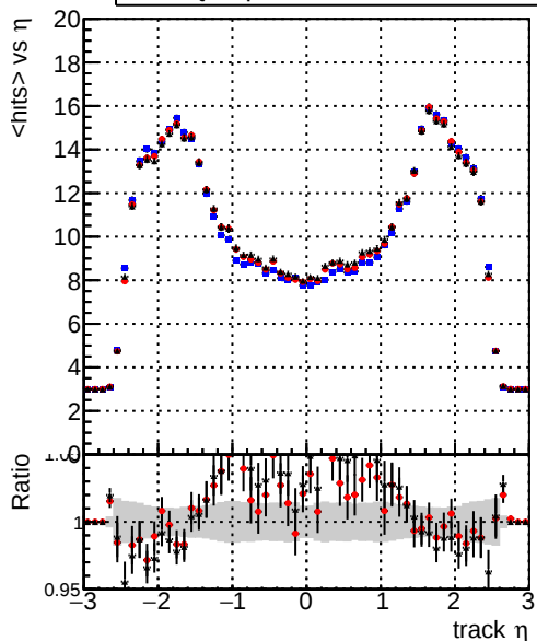
mean hits vs \eta — DQMstep3_TT_CKF — DQMstep3_TT_CKF-t00 — DQMstep3_TT_CKF-t01
