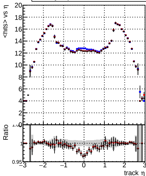
mean hits — DQMstep3_TT_CKF — DQMstep3_TT_CKF-t00 — DQMstep3_TT_CKF-t01
