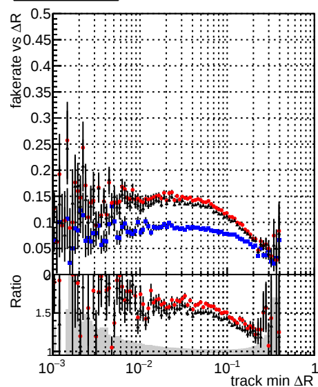
—●— DQMstep3 TT CKF —●— DQMstep3 TT CKF-t00 —●— DQMstep3 TT CKF-t01
