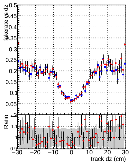
Fake rate vs dz —●— DQMstep3_TT_CKF —●— DQMstep3_TT_CKF-tok
