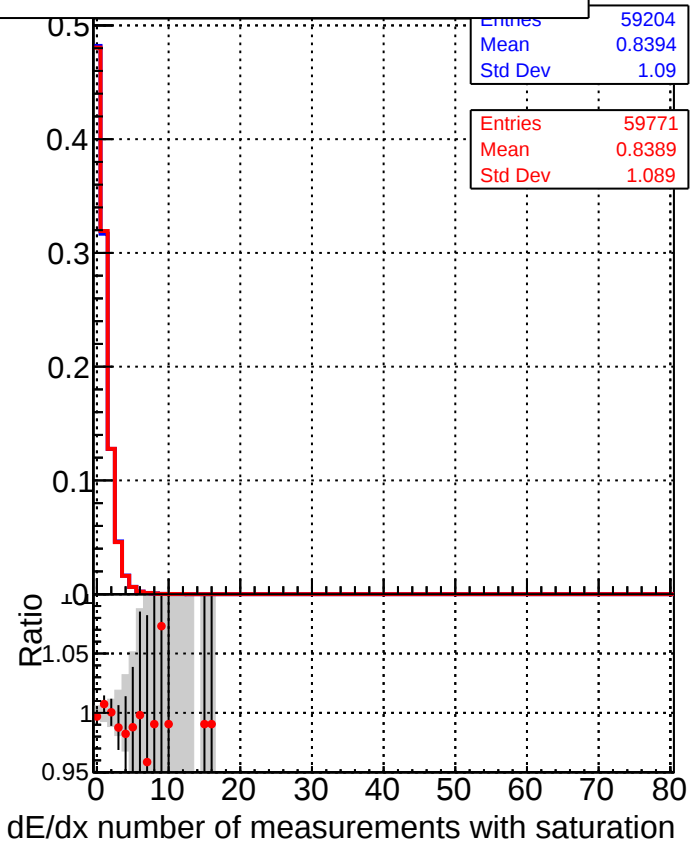
■ DQMstep3_TT_CKF ● DQMstep3_TT_CKF-tok
