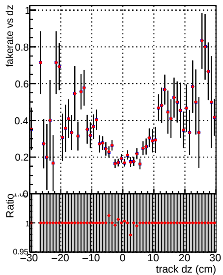
—●— DQMstep3_TT_CKF —●— DQMstep3_TT_CKF-tok
