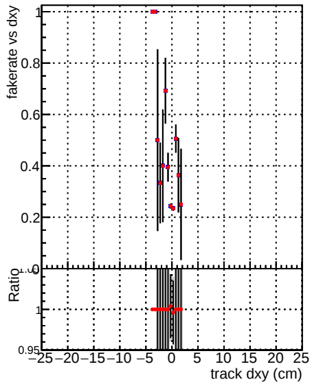
—●— DQMstep3_TT_CKF —●— DQMstep3_TT_CKF-tok
