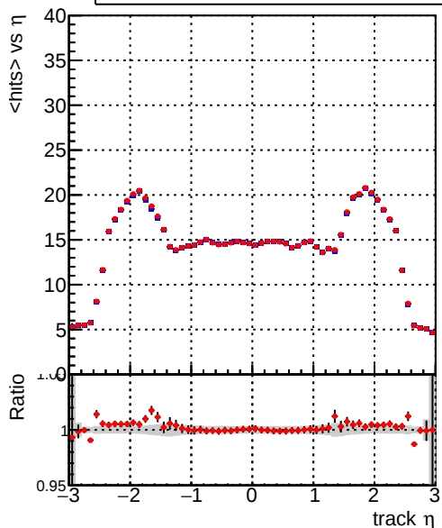
mean hit — DQMstep3_TT_CKF — DQMstep3_TT_CKF-tok
