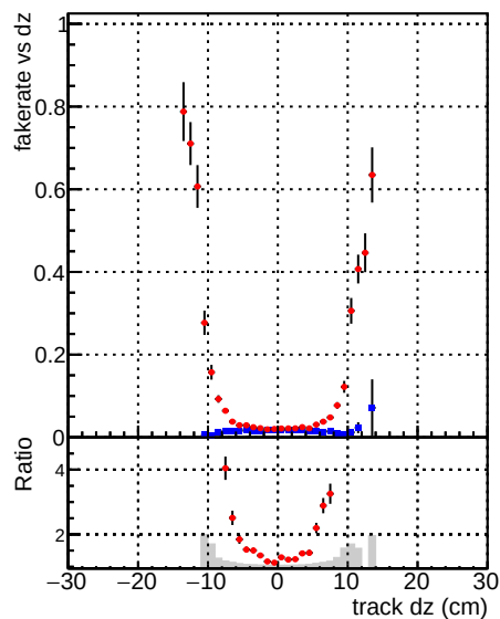
—●— DQMstep3_TT_CKF —●— DQMstep3_TT_CKF-tok
