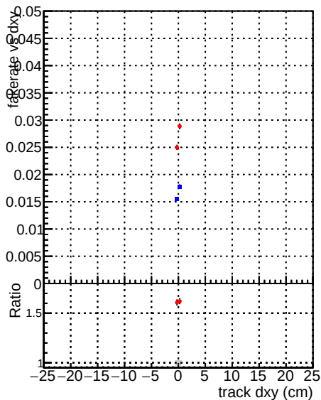
—●— DQMstep3_TT_CKF —●— DQMstep3_TT_CKF-tok
