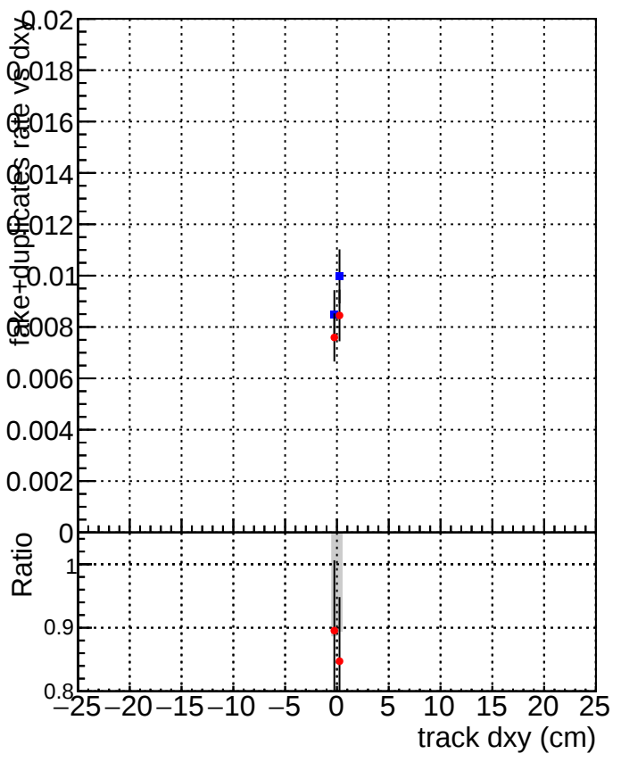
DQMstep3_TT_CKF DQMstep3_TT_CKF-tok
