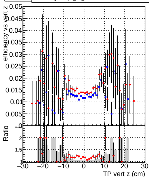
Efficiend —●— DQMstep3_TT_CKF-tok
