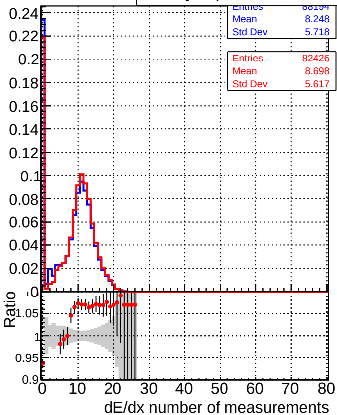
DQMstep3_TT_CKF DQMstep3_TT_CKF-tok
