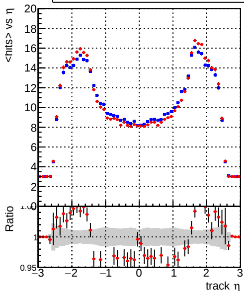
mean hits vs \eta — DQMstep3_TT_CKF — DQMstep3_TT_CKF-tok
