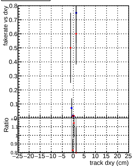
—●— DQMstep3_TT_CKF —●— DQMstep3_TT_CKF-tok
