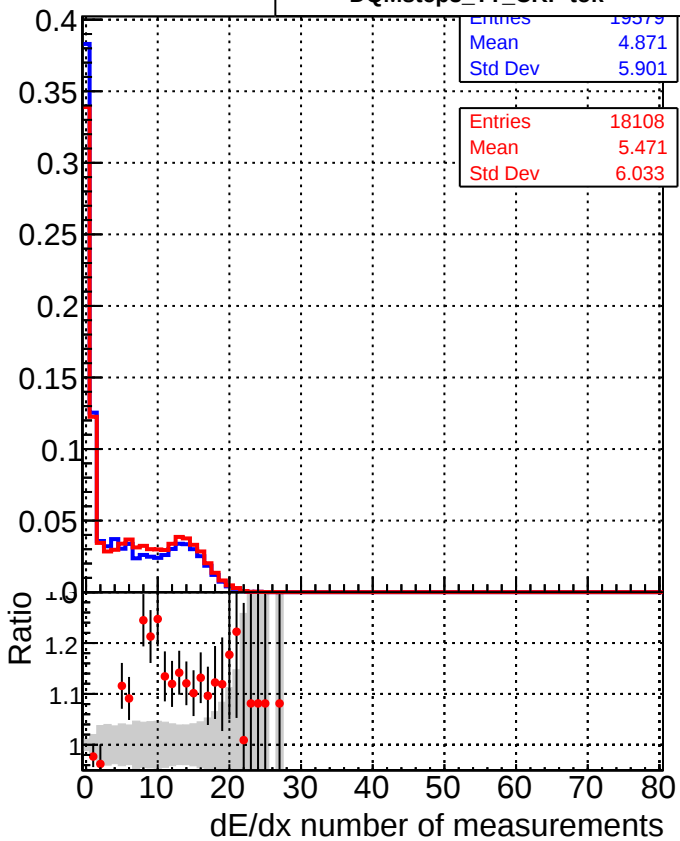
DQMstep3_TT_CKF DQMstep3_TT_CKF-tok
