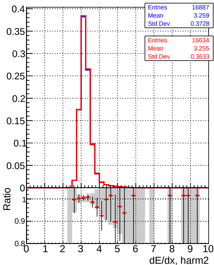
■ DQMstep3_TT_CKF ● DQMstep3_TT_CKF-tok
