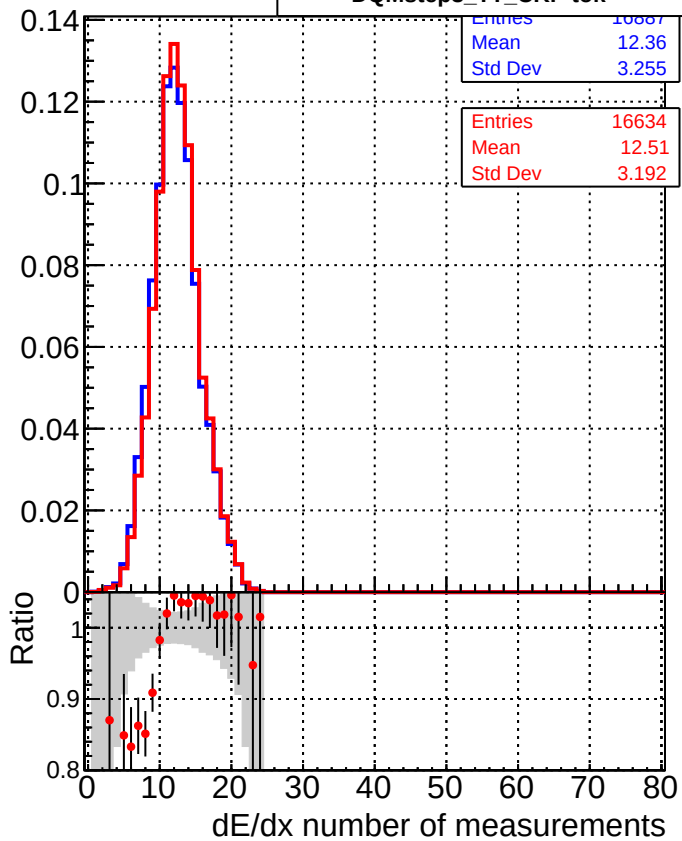
■ DQMstep3_TT_CKF ● DQMstep3_TT_CKF-tok
