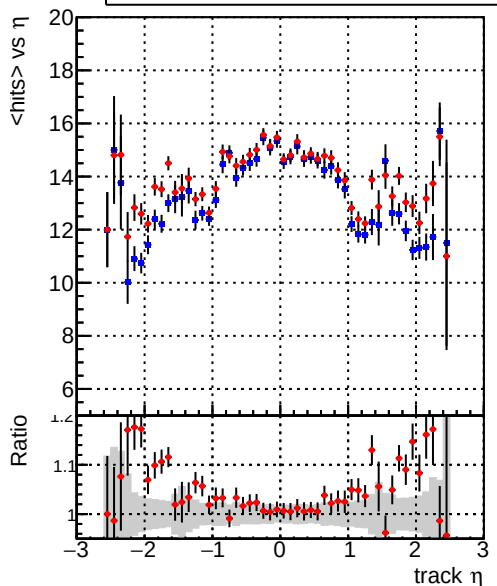
mean hits DQMstep3_TT_CKF DQMstep3_TT_CKF-tok
