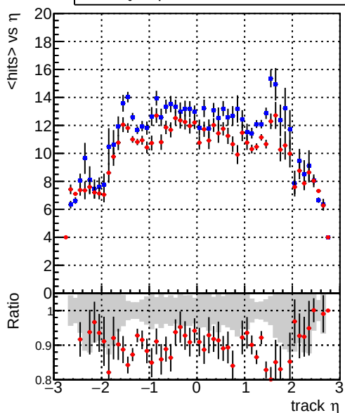
mean hit — DQMstep3_TT_CKF — DQMstep3_TT_CKF-tok
