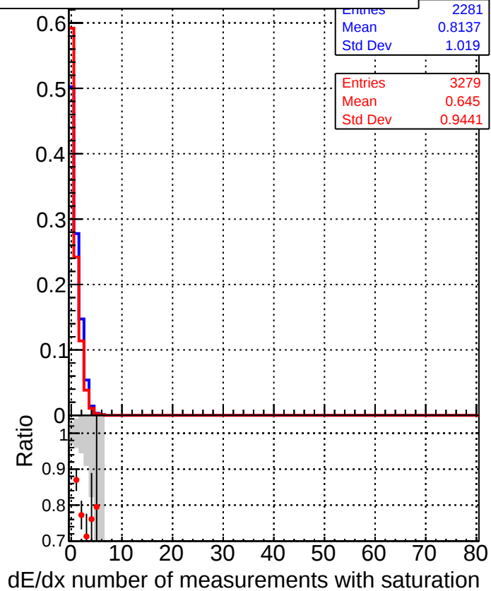
DQMstep3_TT_CKF DQMstep3_TT_CKF-tok
