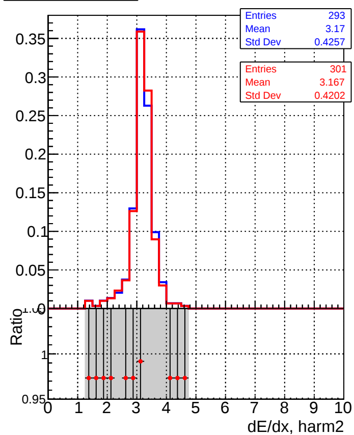
dE/dx estimator 1
