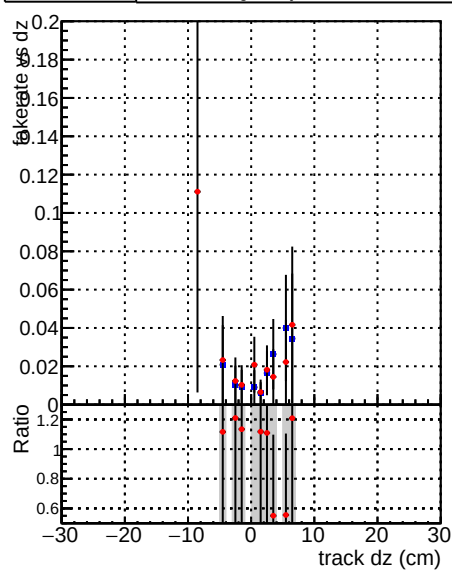
—●— DQMstep3_TT_CKF —●— DQMstep3_TT_CKF-tok
