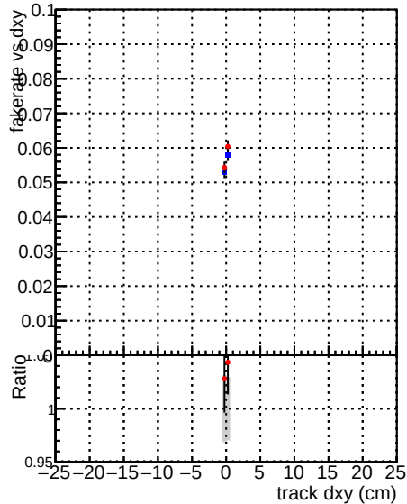
—●— DQMstep3 TT_CKF —●— DQMstep3 TT_CKF-tok
