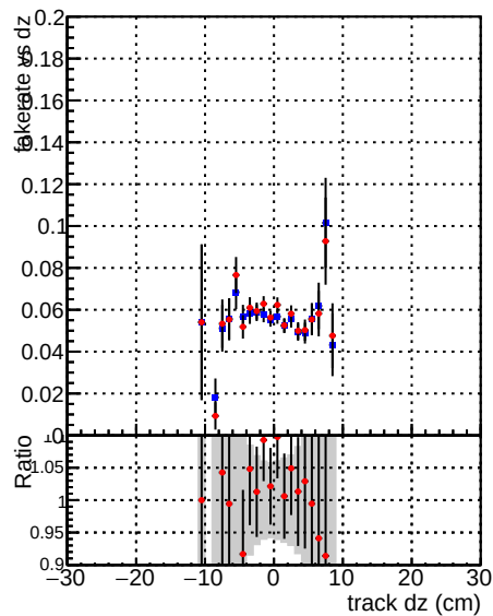
—●— DQMstep3 TT_CKF —●— DQMstep3 TT_CKF-tok
