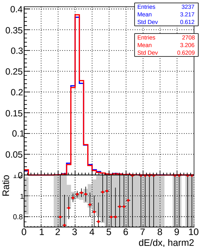
■ DQMstep3_TT_CKF ● DQMstep3_TT_CKF-tok
