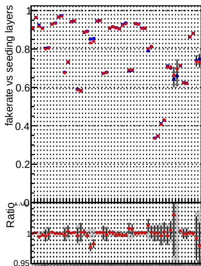
Fake rate vs. DQMstep3 TT_CKF DQMstep3 TT_CKF-tok
