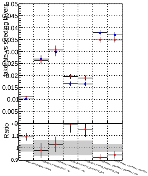
Fake rate vs. —●— DQMstep3 TT_CKF —●— DQMstep3 TT_CKF-tok
