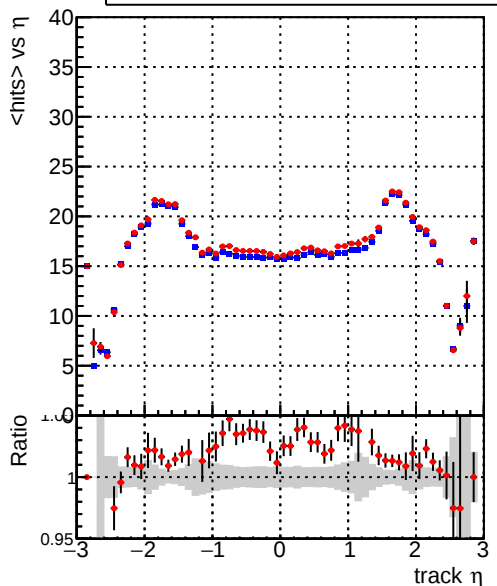
mean hit — DQMstep3_TT_CKF — DQMstep3_TT_CKF-tok
