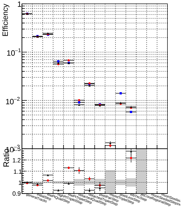
DQMstep3_TT_CKF DQMstep3_TT_default DQMstep3_TT_defaultNEWT
