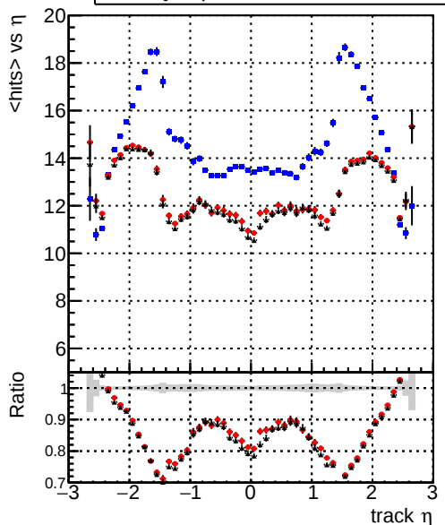
mean hits vs \eta — DQMstep3_TT_CKF — DQMstep3_TT_default — DQMstep3_TT_defaultNEWT
