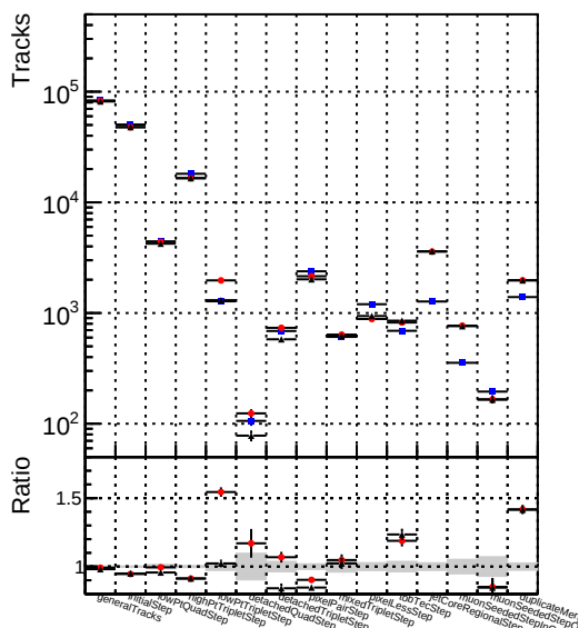
—●— DQMstep3_TT_CKF —●— DQMstep3_TT_default —●— DQMstep3_TT_defaultNEWT
