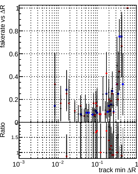
Fake rate vs \Delta R(\text{track, jet}) DQMstep3 TT CKF DQMstep3 TT default DQMstep3 TT defaultNEWT
