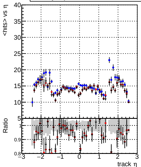
mean hit — DQMstep3_TT_CKF — DQMstep3_TT_default — DQMstep3_TT_defaultNEWT
