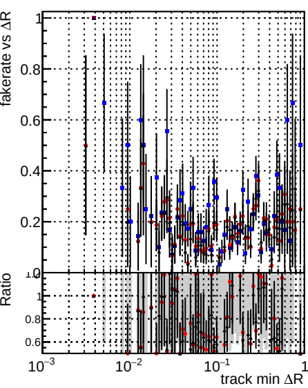
Legend: DQMstep3 TT CKF (blue dots), DQMstep3 TT default (red dots), DQMstep3 TT defaultNEWT (black dots)
