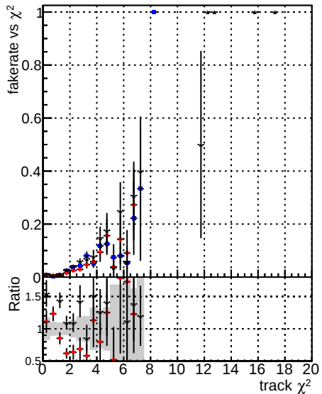
Fake rate vs. DOMstep3 TT CKF DOMstep3 default DOMstep3 defaultNEWT
