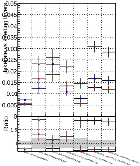
Fake rate vs. DOMstep3 TT CKF DOMstep3 default DOMstep3 defaultNEWT
