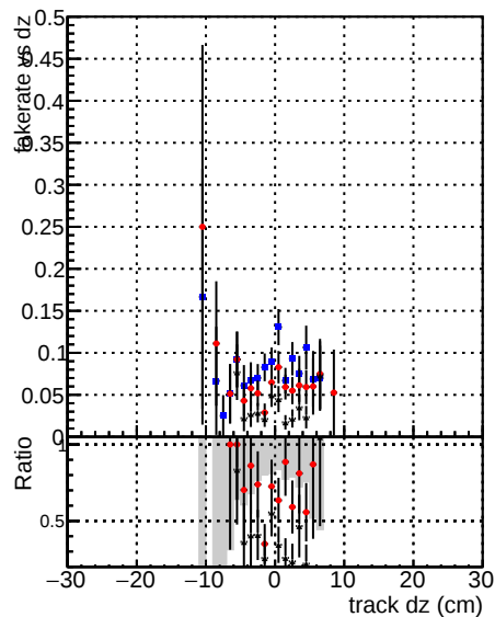
Fake rate vs dz DOMstep3 TT CKF DOMstep3 default DOMstep3 defaultNEWT
