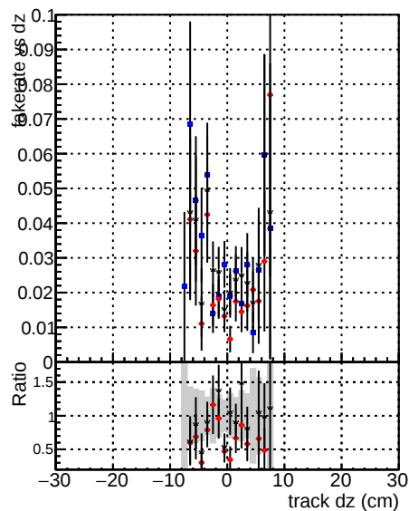
Fake rate vs dz DOMstep3 TT CKF DOMstep3 TT default DOMstep3 TT defaultNEWT
