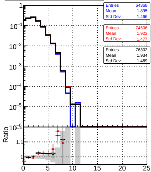
mean hit — DQMstep3_TT_CKF — DQMstep3_TT_default — DQMstep3_TT_defaultNEWT
