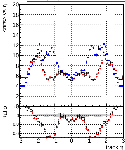
mean hits — DQMstep3_TT_CKF — DQMstep3_TT_default — DQMstep3_TT_defaultNEWT
