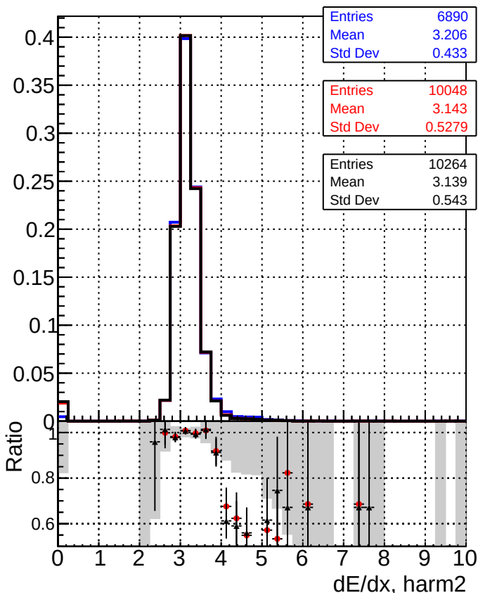
—■ DQMstep3_TT_CKF —● DQMstep3_TT_default —■ DQMstep3_TT_defaultNEWT
