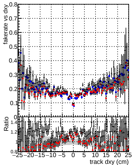
—●— DOMstep3 TT CKF —●— DOMstep3 default —●— DOMstep3 defaultNEWT2
