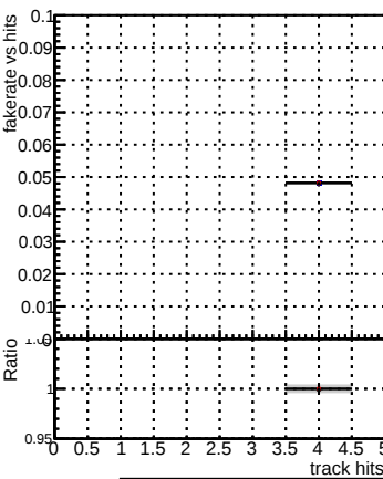
Fake rate vs hit Legend: DQMstep3_TT_CKF DQMstep3_TT_default DQMstep3_TT_defaultNEWT2
