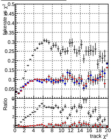
Fake rate vs. — DOMstep3 TT GKF — DOMstep3 default — default NEWT2
