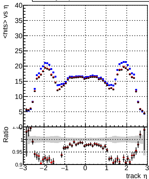
— DQMstep3_TT_CKF — DQMstep3_TT_default — DQMstep3_TT_defaultNEWT2 mean hits
