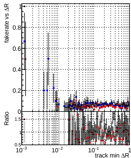
Legend: DQMstep3 TT CKF (blue squares) DQMstep3 TT default (red circles) DQMstep3 TT defaultNEW2 (black crosses)
