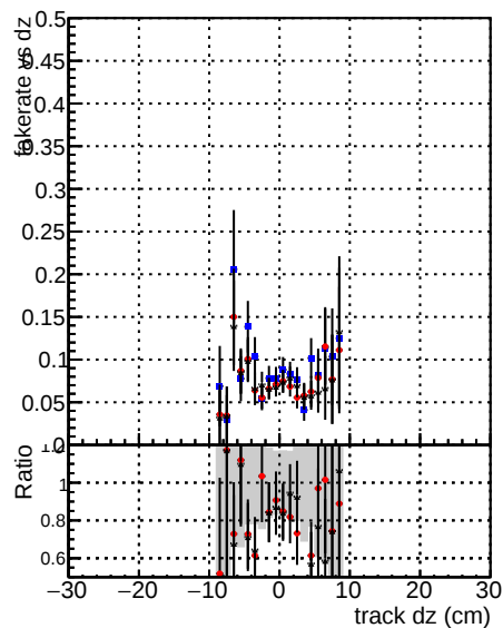
Fake rate vs d —●— DOMstep3 TT CKF —●— DOMstep3 TT default —●— DOMstep3 TT defaultNEW2
