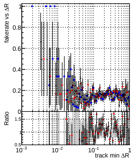
—●— DQMstep3_TT_CKF —●— DQMstep3_TT_default —●— DQMstep3_TT_defaultNEW2
